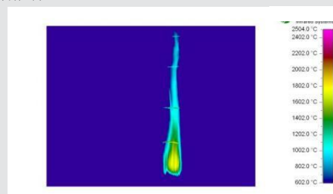
PYROVIEW640C 火焰热图像
