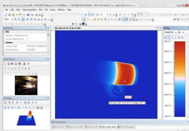
PYROVIEW 640F 透过火焰测温成像
